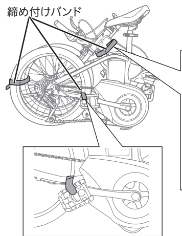
⑥付属の締め付けバンド(3本)で、前後の車輪、ハンドル、ペダルとチェーンステアを結束する
